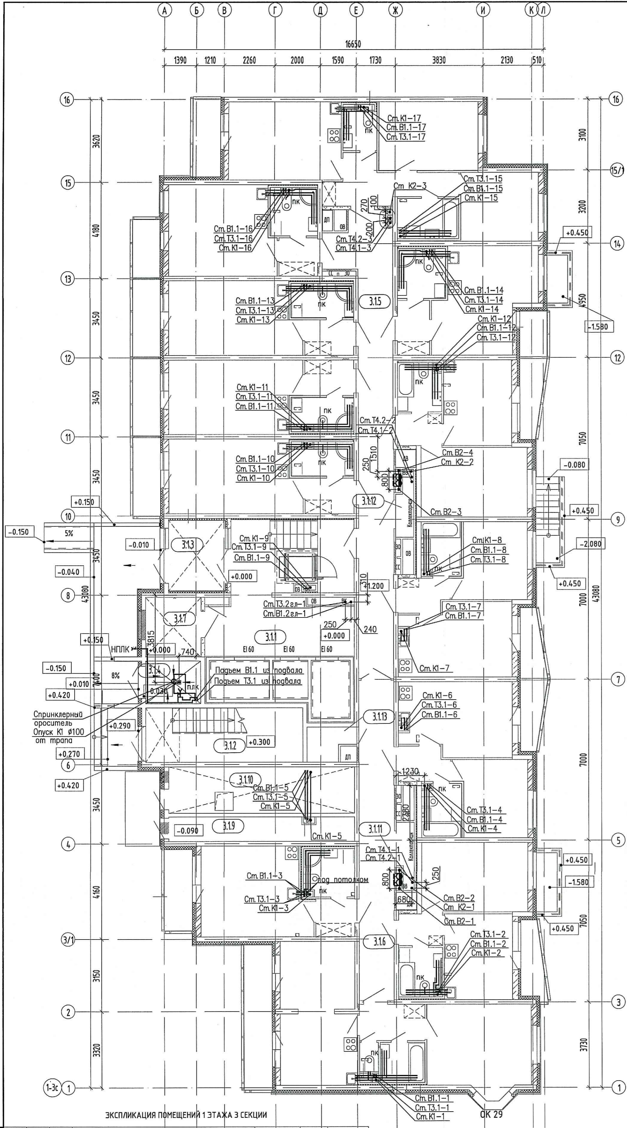
Схема расположения секции
